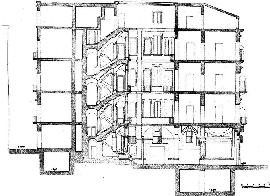
Napoli, palazzo Mastellone. Sezione tra piazza Salvo d'Acquisto e via Simonelli.
